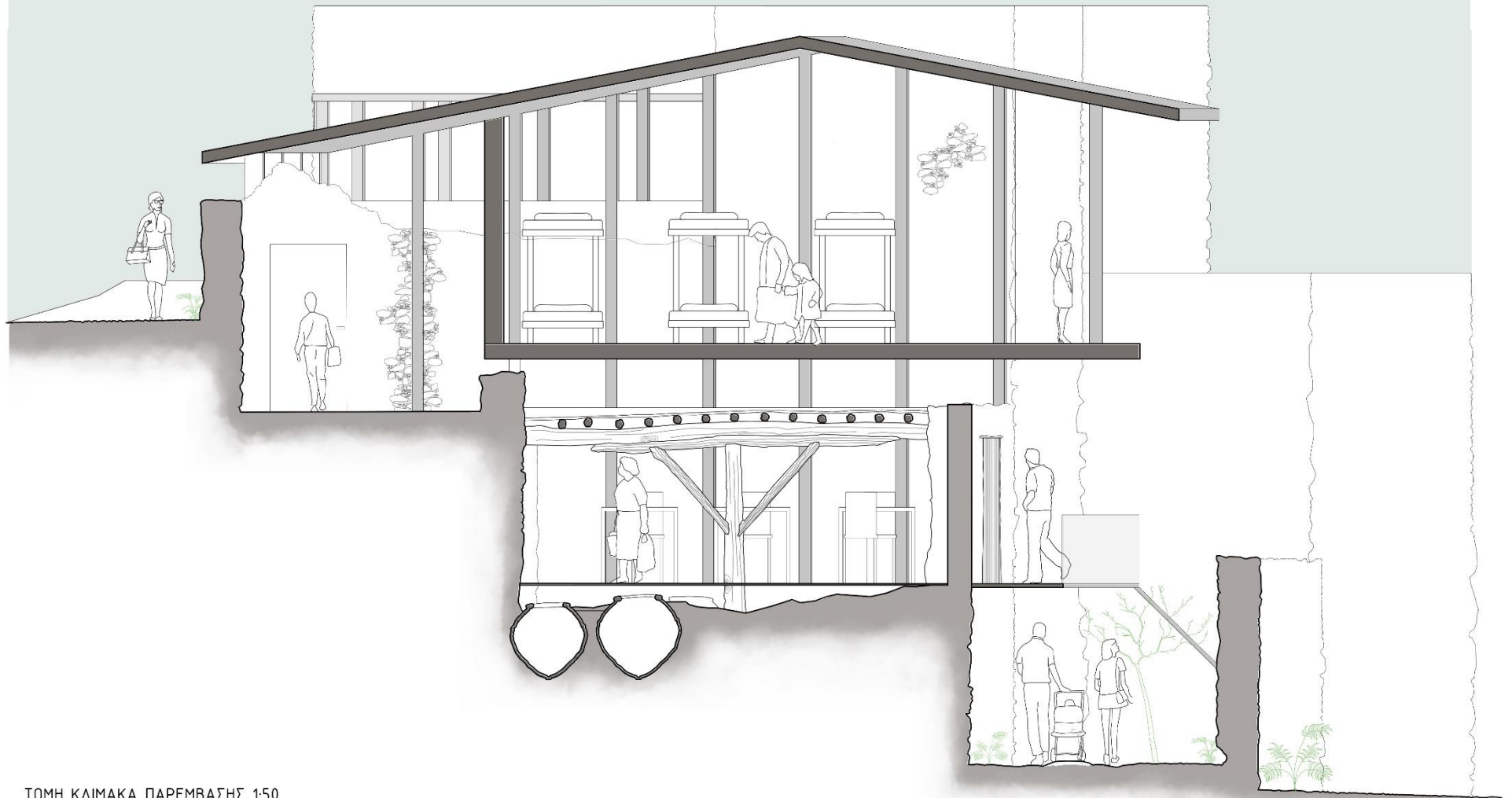
ΤΟΜΗ ΚΛΙΜΑΚΑ ΠΑΡΕΜΒΑΣΗΣ 1:50
