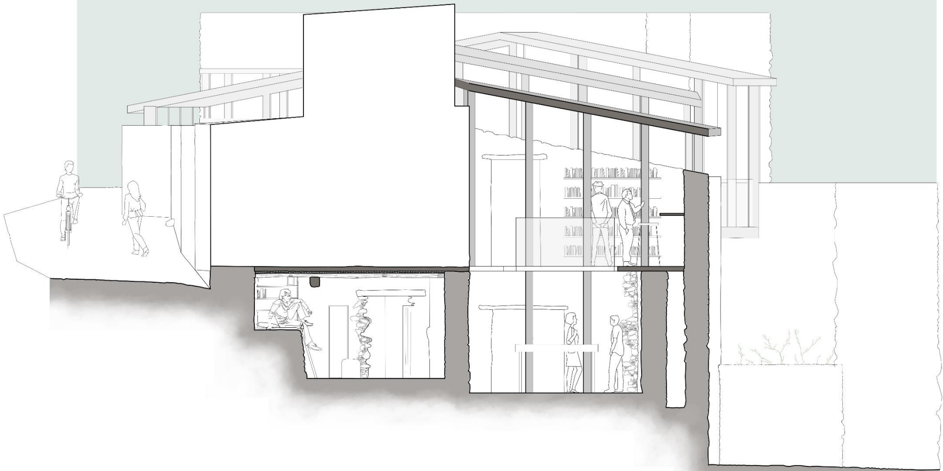
ΤΟΜΗ ΚΛΙΜΑΚΑ ΠΑΡΕΜΒΑΣΗΣ 1:50
